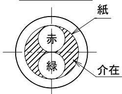
コード断面図
