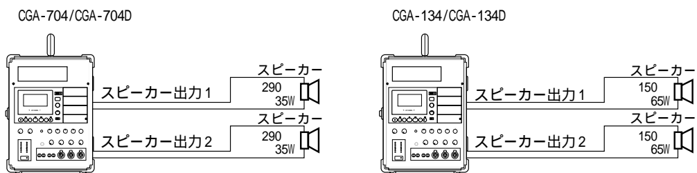
図2 接続例
