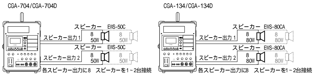
図1 接続例
