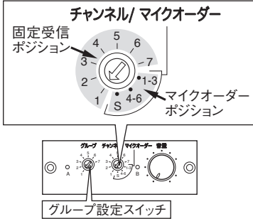
チャンネル設定スイッチ
