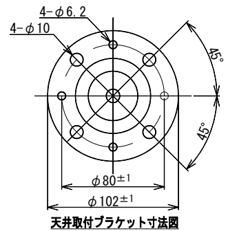
天井取付ブラケット寸法図
