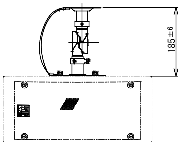
HMB-80HA横取付時
