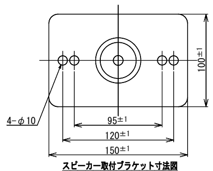
スピーカー取付ブラケット寸法図
