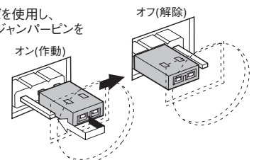
図4 ①ゴムキャップを取り外す ②内部のジャンパーピンを差し換える
